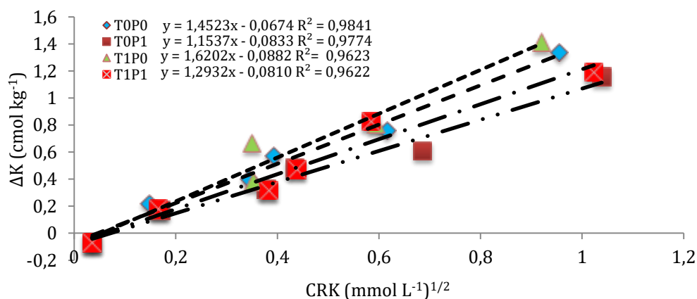
Gambar 1. Kurva Quantity-Intensity (Q/I) Kalium di Tanah Ultisol Gedung Meneng Sebelum Tanam pada Musim Tanam Kesembilan ; TOP0 (Olah Tanah Minimum +Pemupukan Setengah), TOP1(Olah Tanah Minimum+ Pemupukan Penuh), T1P0 (Olah Tanah Intensif+Pemupukan Setengah), T1P1 (Olah Tanah Intensif+Pemupukan Penuh); CR_K : Konsentrasi rasio; \Delta K : Jumlah K yang dijerap atau pelepasan K dari tanah
