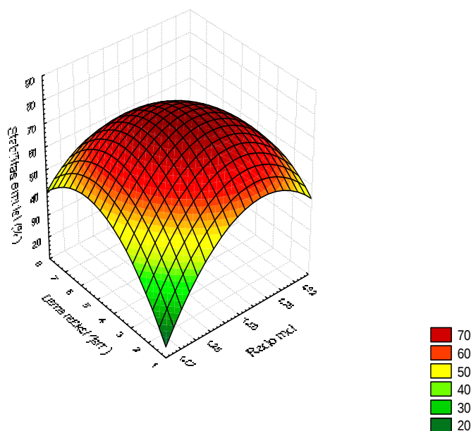
Gambar 4. Permukaan respon nilai stabilitas emulsi sebagai fungsi dari lama reaksi dan rasio mol pada MES
