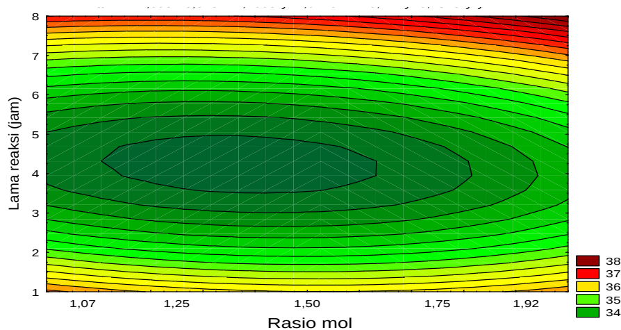
Gambar 3 Kontur respon nilai tegangan permukaan sebagai fungsi dari rasio mol reaktan dan lama reaksi pada MES
