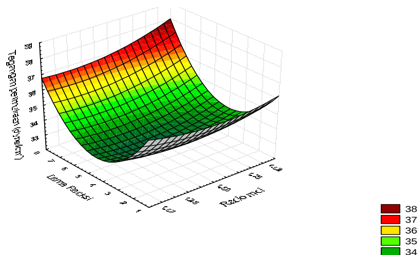
Gambar 2 Permukaan respon nilai tegangan permukaan sebagai fungsi dari rasio mol reaktan dan lama reaksi pada MES
