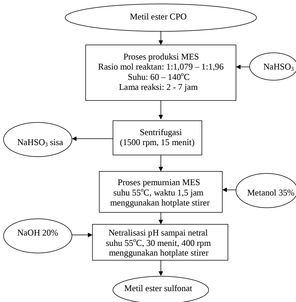
Gambar 1 Diagram alir proses produksi MES dari metil ester CPO menggunakan NaHSO 3 (modifikasi Sheats dan Mac Arthur, 2002).
